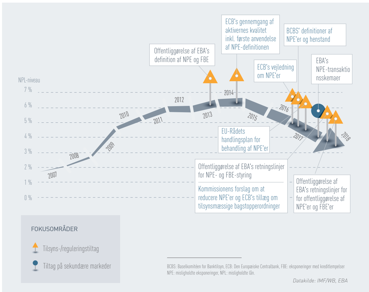
Figur 3: Misligholdte lån (NPL'er) i EU — på vej mod genopretning
